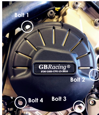
Bolt 4 M6X30TORX - 8Nm
