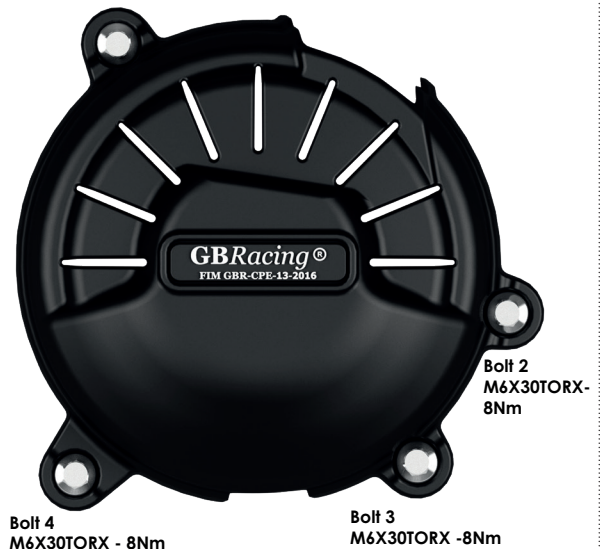
Bolt 1 M6X30TORX - 8Nm
